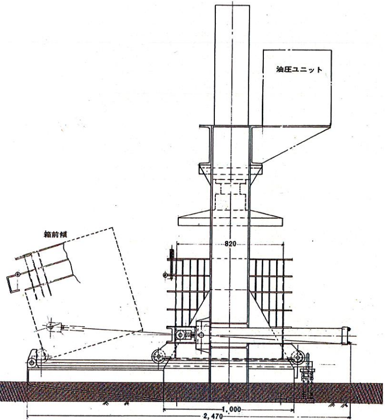
●側面図
