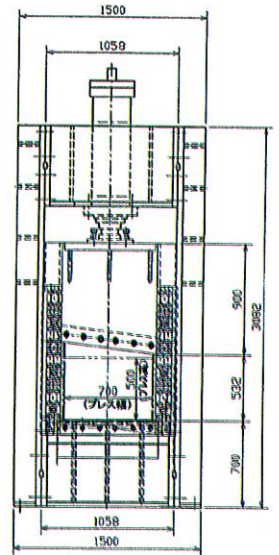
●正面図
