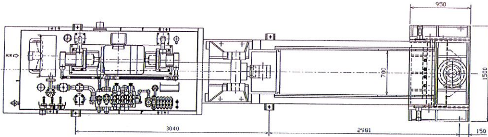
●上面図
