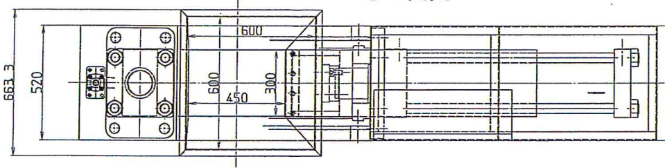
●上面図
