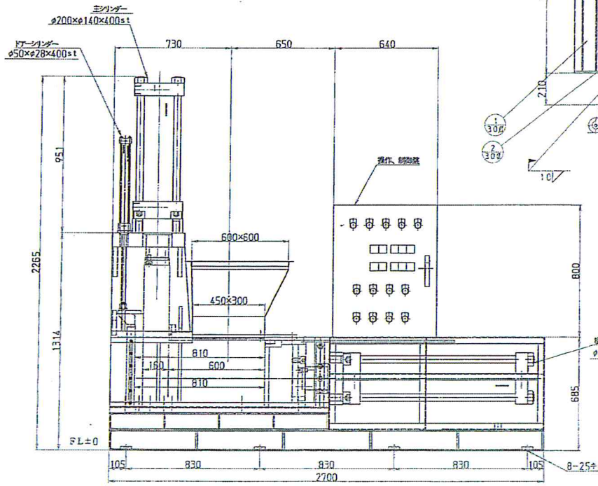
●側面図
